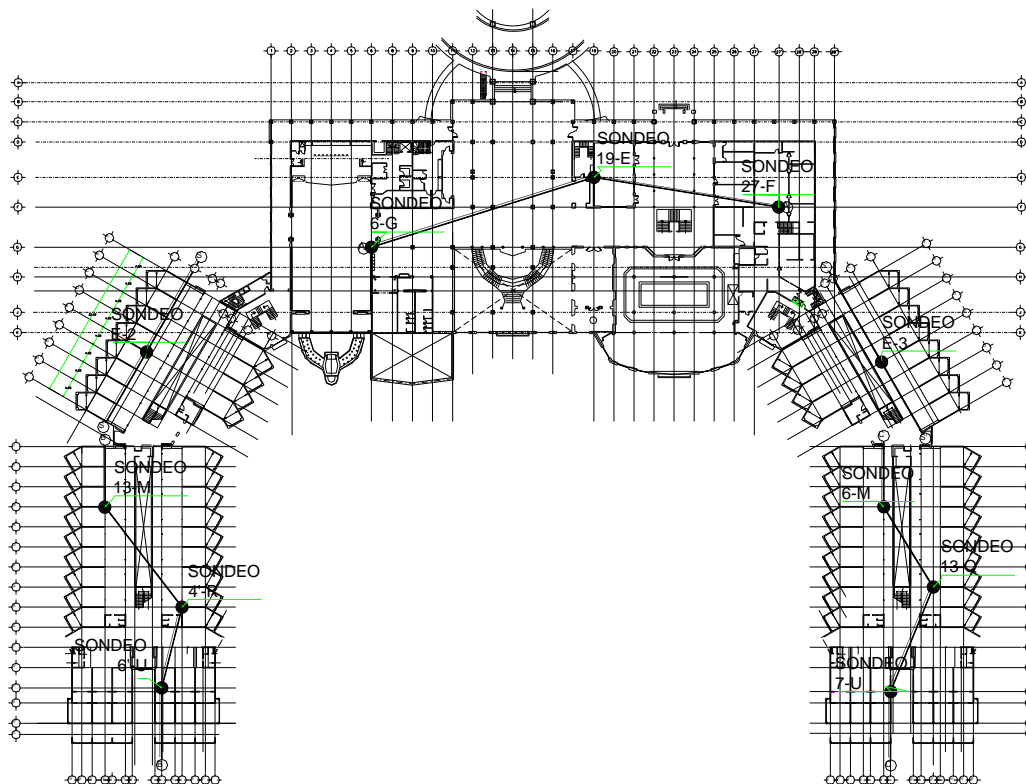
Figura 2, Ubicación de sondeos mecánicos en el Hotel Capri Caribe Secrets, en Playa del Carmen. Q.R.
