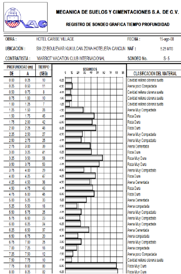
Figura 3. Perfil estratigráfico típico de un sondeo realizado con avance controlado
